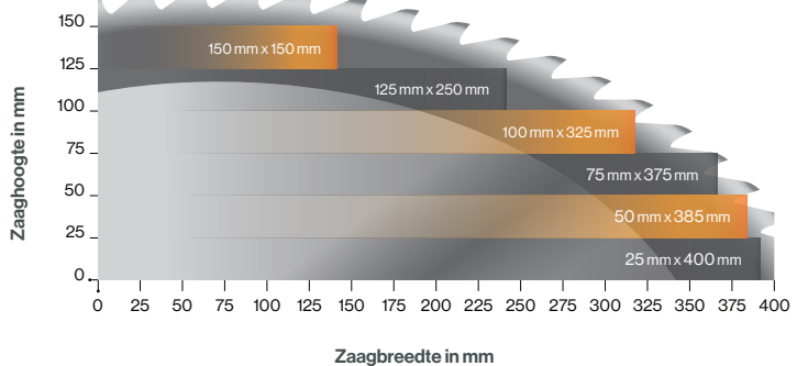
TigerSaw1000 - Zaagbereik Zaagblad: 500 mm
