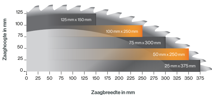
TigerSaw1000 - Zaagbereik Zaagblad: 450 mm
